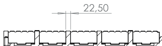
COUPE A-A
